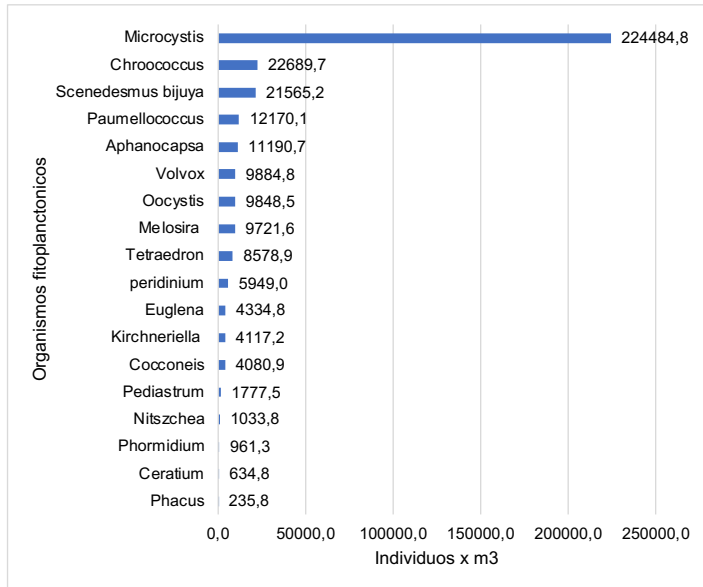
Figura 3. Representación gráfica de organismos fitoplanctónicos identificados en el tercer muestreo de la laguna en estudio.
