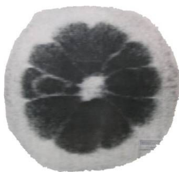
Figura 9. Primera imagen RMI realizada en limón (Hinshaw, 1977).
