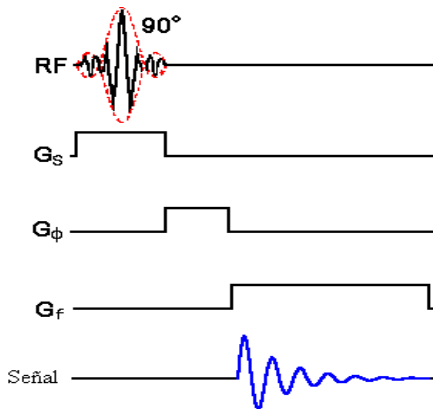
Figura 8. Secuencia simplificada de reconstrucción de una imagen FT bidimensional.
