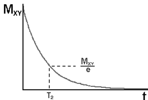
Figura 5. Relajación transversal T_2 .
