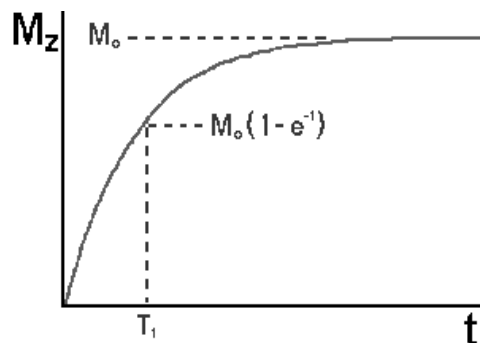
Figura 4. Relajación longitudinal T_1 .
