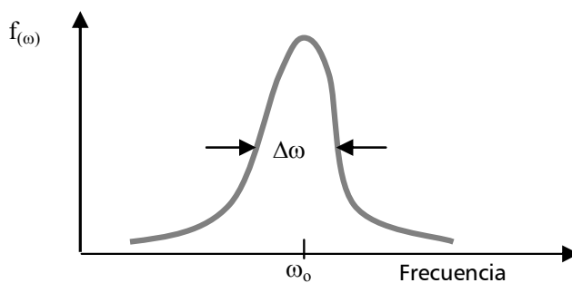
Figura 6. FT de la señal de FID.
