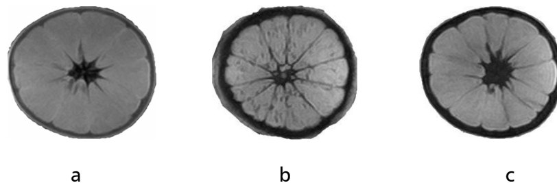
Figura 11. Imágenes RMI de daños internos en naranja producidos por los hongos: a. Alternaria citri , b. Diplodia natalensis , c. Botrytis cinerea (Aristizábal, 2006).
