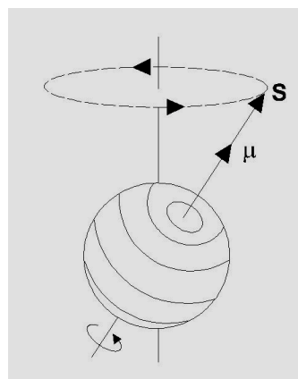
Figura 1. Momentos resultantes sobre un protón.
