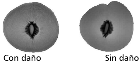
Figura 13. Imágenes RMI del daño por frío en melocotón (Aristizábal 2006).
