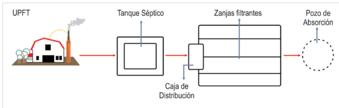
FIGURA 51. Sistema para la disposición de aguas residuales.
