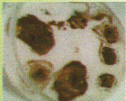
Figura 2. Gránulos de suelo (izquierda) y aislamientos de Azotobacter spp (Derecha).
