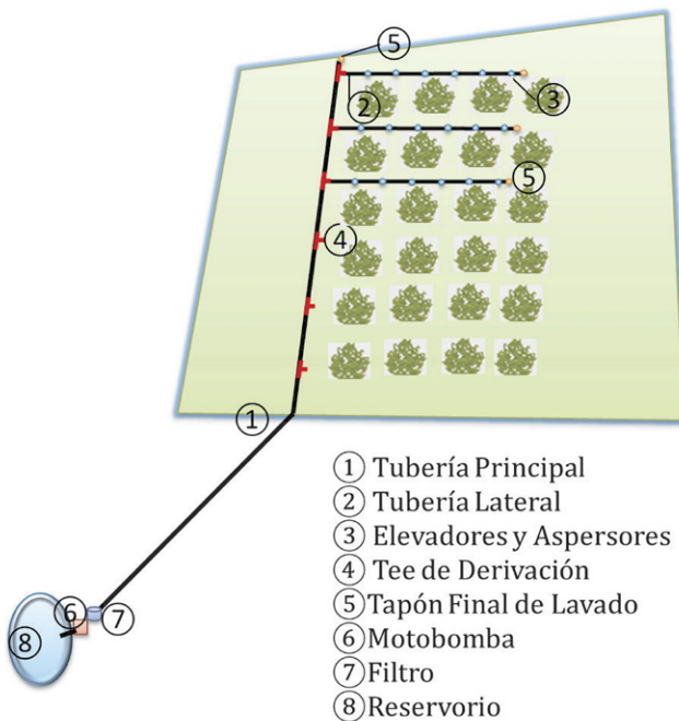
Figura 7 Diseño del sistema de riego por aspersión establecido en la PIPA de Nemocón. Fuente: Equipo CTA-2 Subproyecto Hortalizas (2018).
