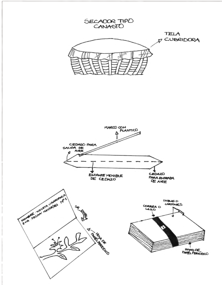
Secador canasta
