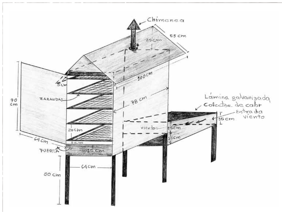
Secador solar
