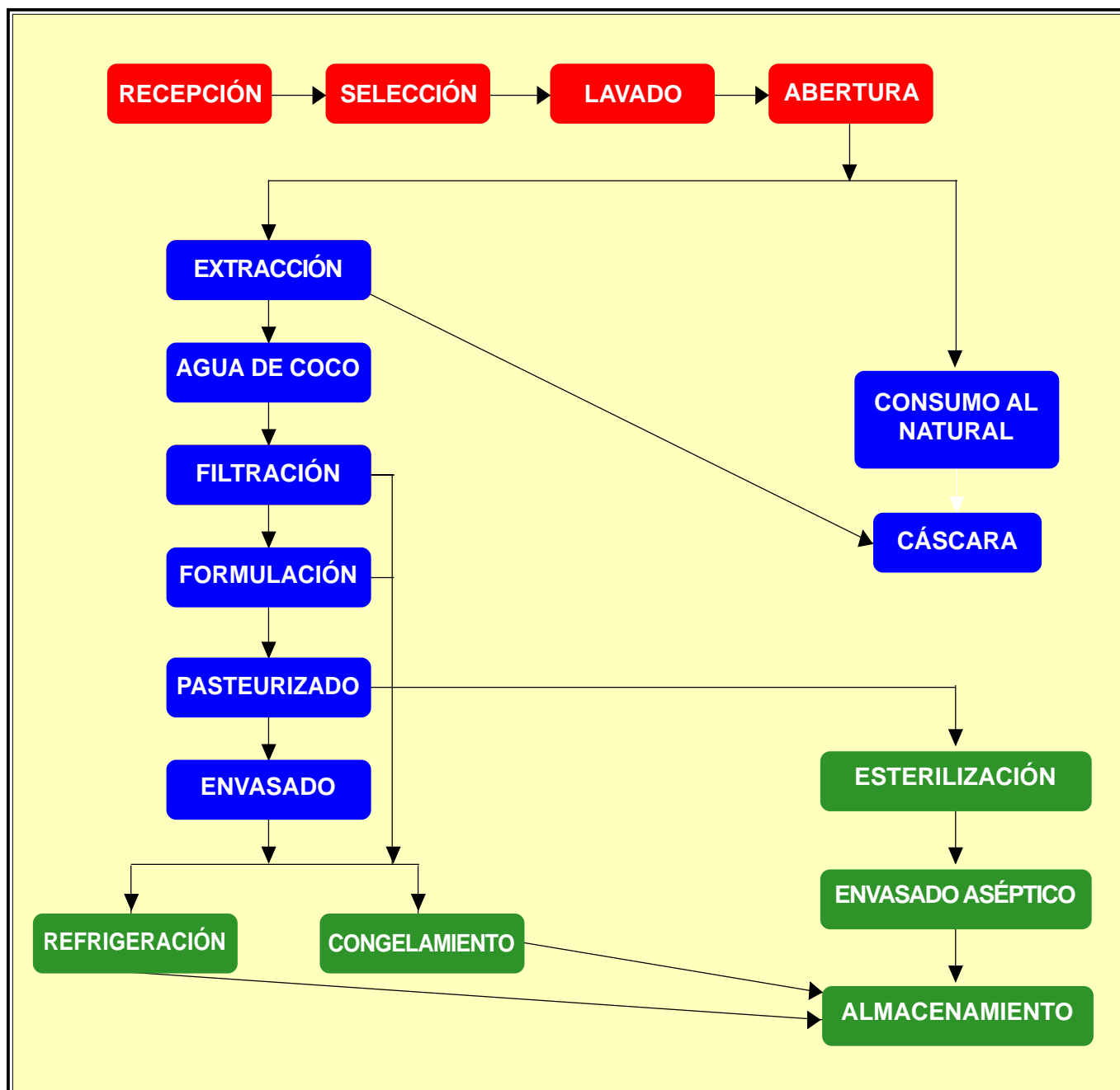
Figura No. 14: Etapas del Proceso de Conservación del Agua de Coco
