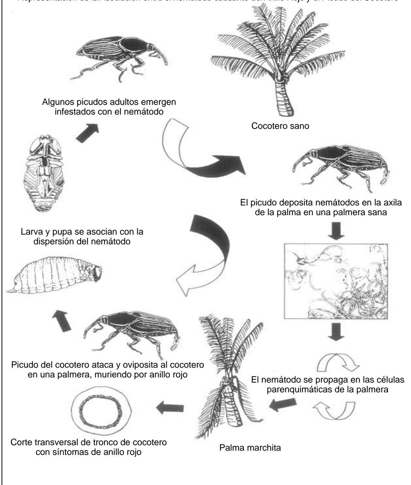
Figura No. 11: Ciclo de Transmisión de la Enfermedad del Anillo Rojo Representación de la Asociación entre el nemátodo causante del Anillo Rojo y el Picudo del Cocotero
