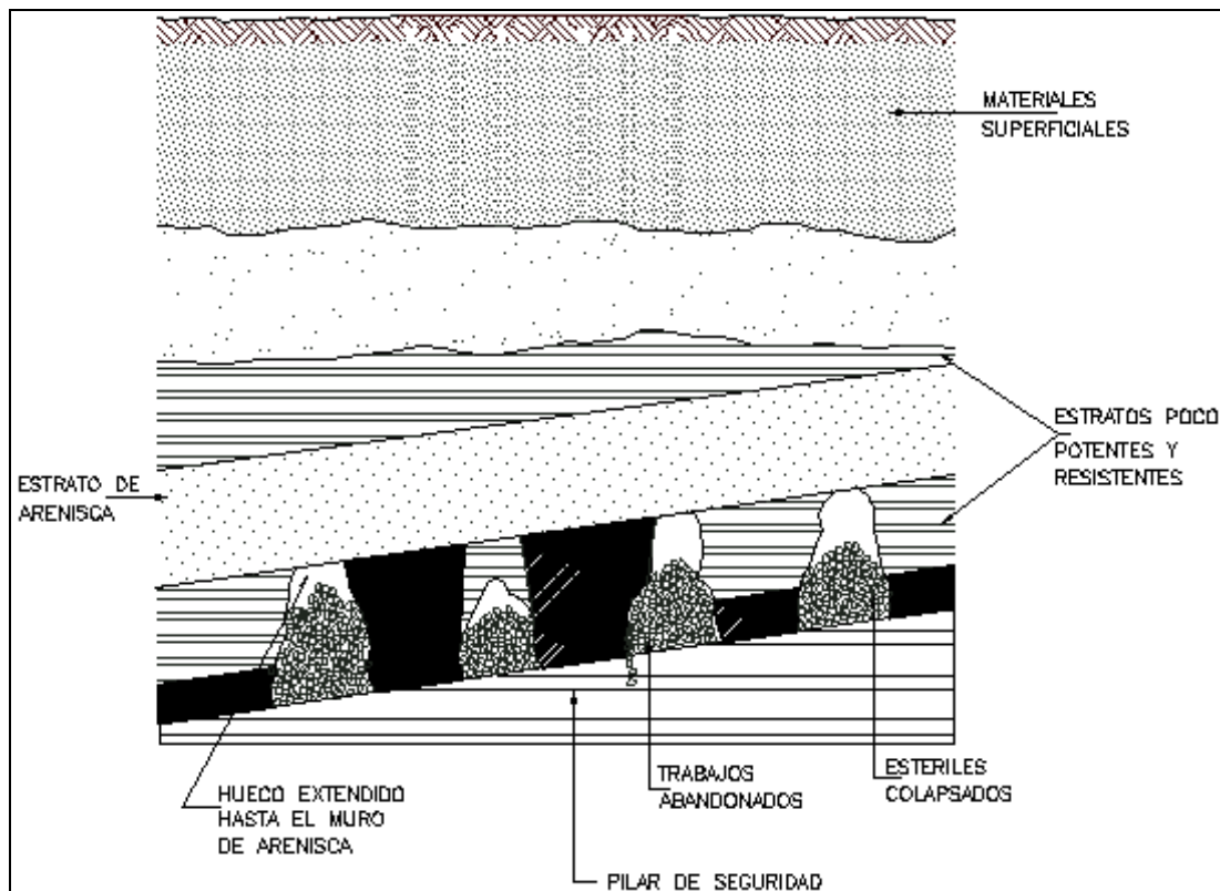
Figura 7.15. Pilares de seguridad
