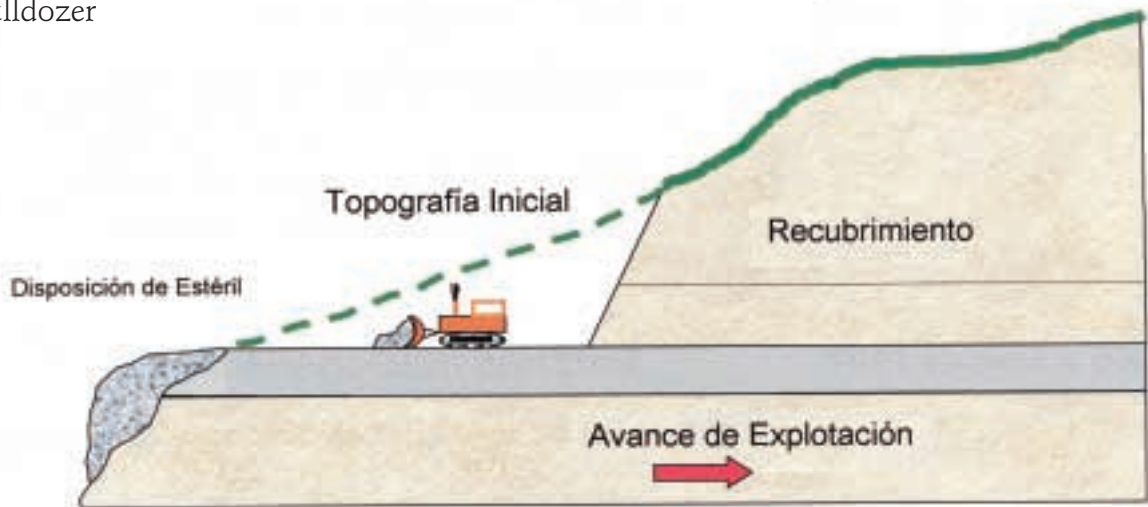
Figura. 5.5 Minería de Contorno
