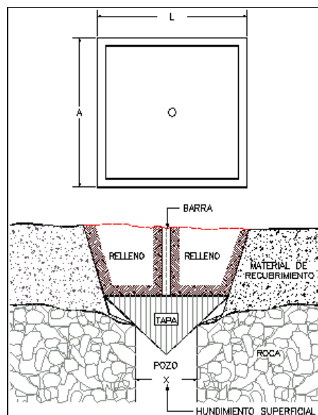
Figura 7.18 Extracción parcial
