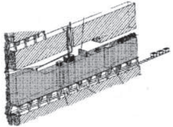
Figura. 5.9 Método de Explotación Tajo Largo. Se aprecia la guía y la galería de explotación. Fuente: Fundamentos de Laboreo de Minas.
