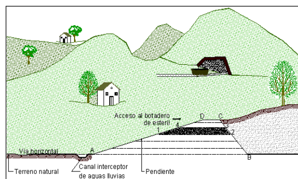
Figura 7.22. Conformación de escombreras por apilamiento en extremos
