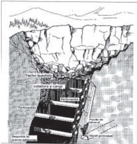
Figura 5.11 Explotación de derrumbe. Fuente: Fundamentos de Laboreo de Minas
