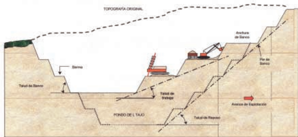
Figura. 5.3 Método de Explotación o Tajo Abierto
