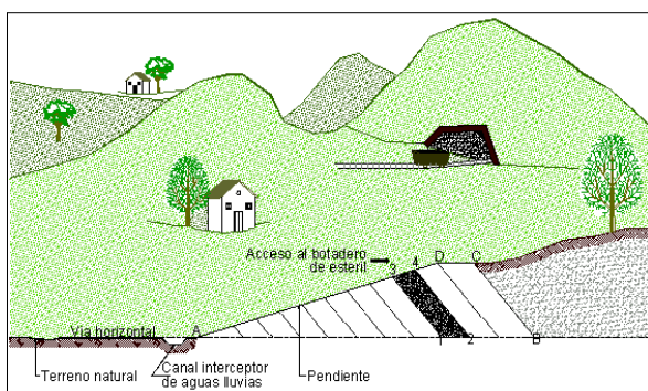
Figura 7.21. Conformación de escombreras por apilamiento en capas
