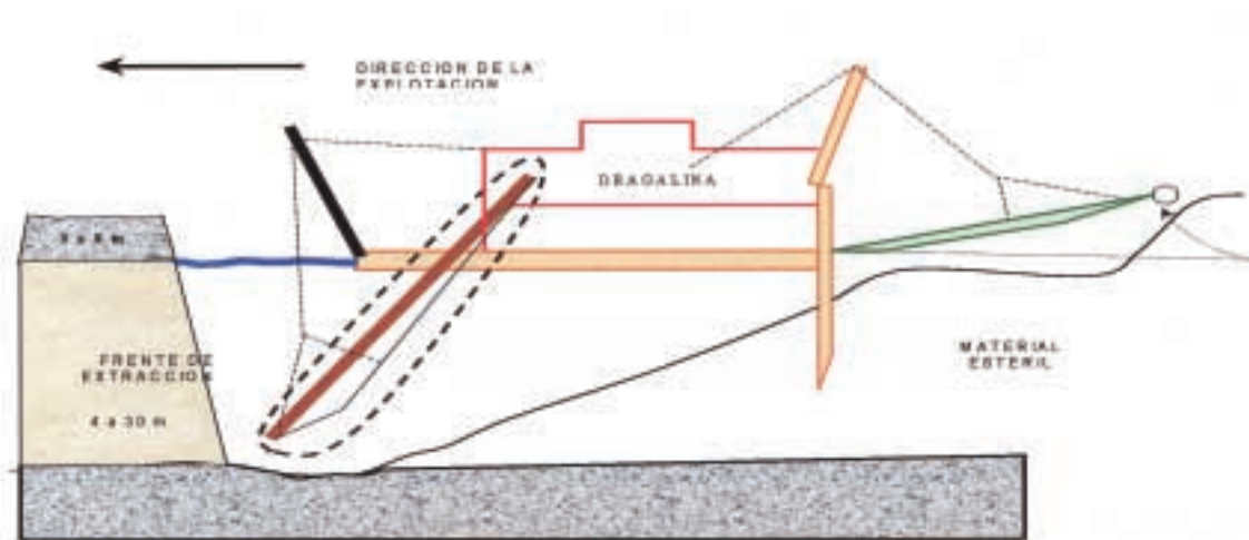
Figura 5.7. Minería de Dragado en Aluviones.
