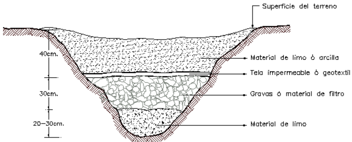
Figura 7.8. Sellamientos y cubrimientos. Fuente: ECOCARBON, 1997.
