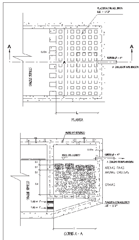
Figura. 7.6 . Filtro anaeróbico
