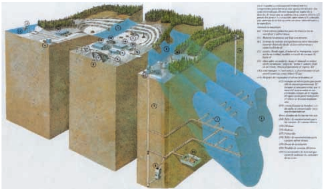
Figura 5.2 Bloque diagrama de explotación a cielo abierto y subterráneo. Fuente: Placer DOME INC- Proceso de Desarrollo de una Mina.
