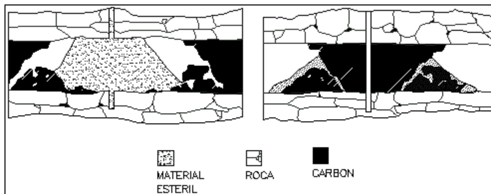
Figura 7.16. Retrollenado
