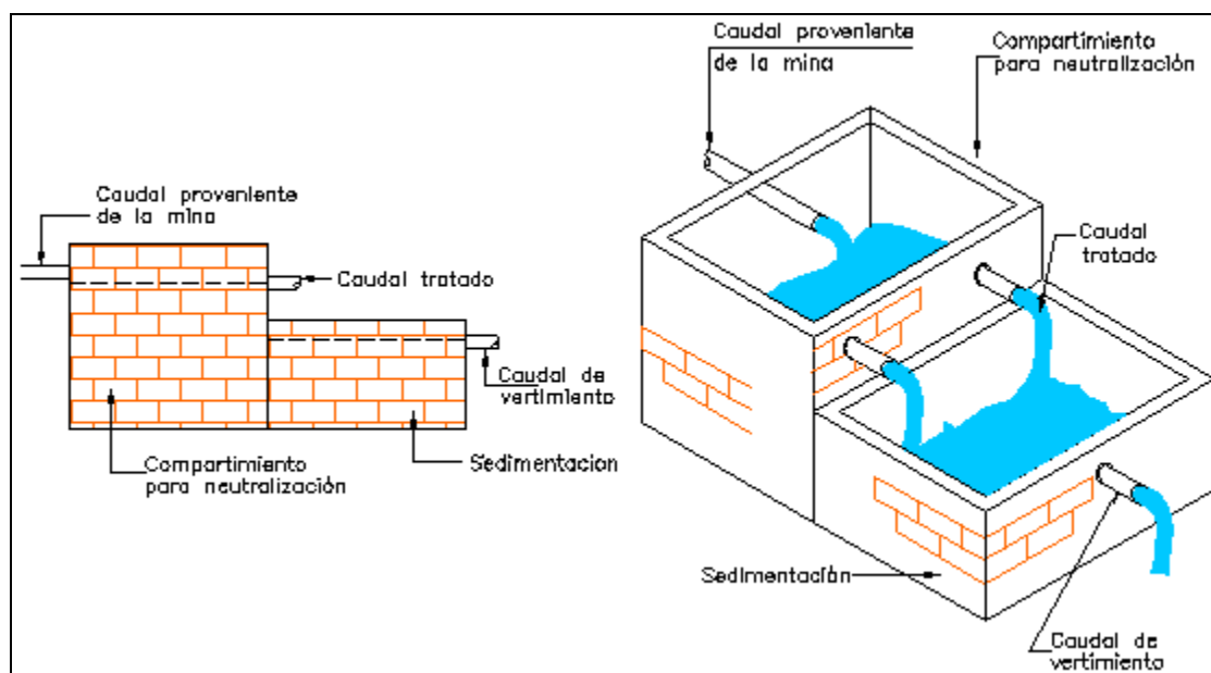
Figura 7.10. Tanques de neutralización. Fuente: ECOCARBON, 1997.
