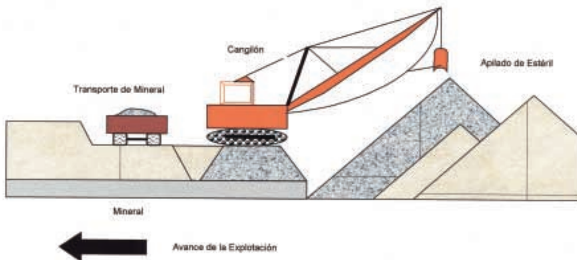
Figura. 5.4 Minería de Cajón o Descubiertas
