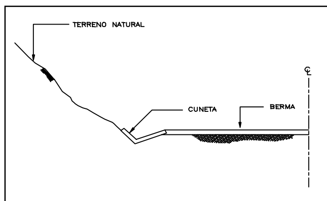
Figura 7.23 Adecuación de accesos.
