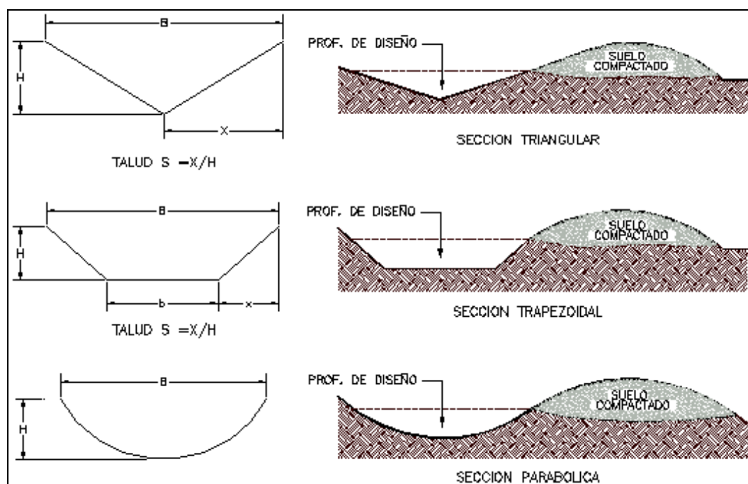
FIGURA 7.7 Interceptación de aguas por canales
