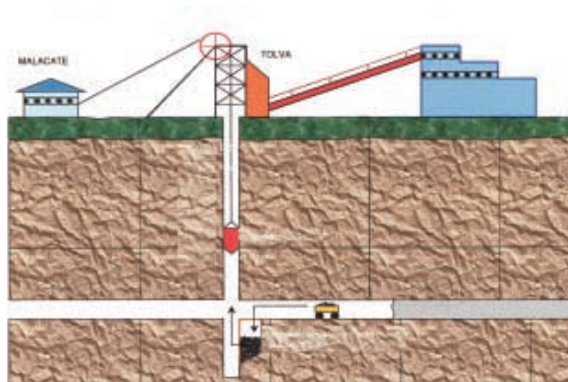
Figura 5.12. Sistema de extracción de mineral mediante malacate y almacenamiento fuera de mina. Fuente: Tomado y modificado de Introducción a la Geología y Minería al Carbón para Ingenieros
