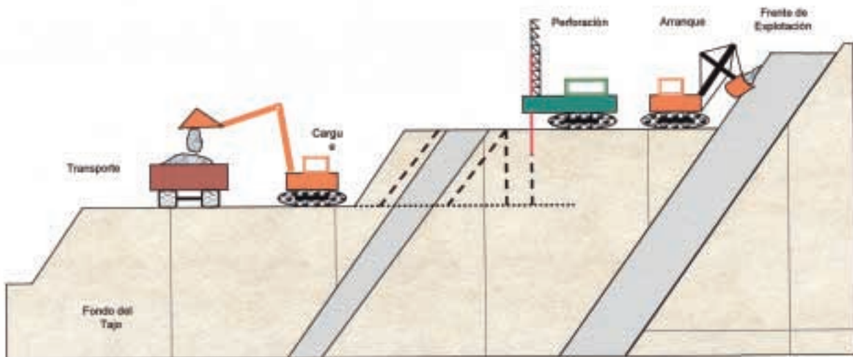
Figura. 5.6 Minería de Tajo Largo
