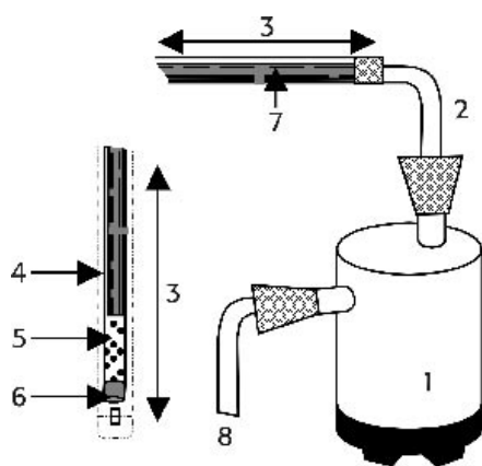
Figura 1: Montaje y sonda utilizados en la recuperación microbiana: 1) Recipiente de recolección, 2) Conexión a la sonda a introducir en el rumen, 3) Sonda (va al rumen), 4) Cubierta plástica temporal, 5) Agujeros, 6) Tapón, 7) Soporte interno de la sonda y 8) Conexión a la bomba de succión.
